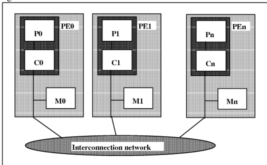
Fig.1.4. The COMA Model
