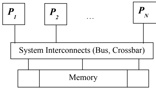
Fig.1.2. The UMA Model
